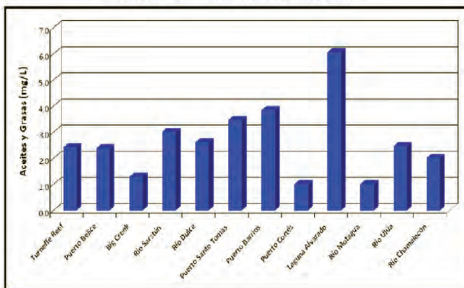
Figura 3.2-29. Campaña de Prospección Ambiental: Matriz "Agua" – Mediciones de laboratorio: Aceites y Grasas
